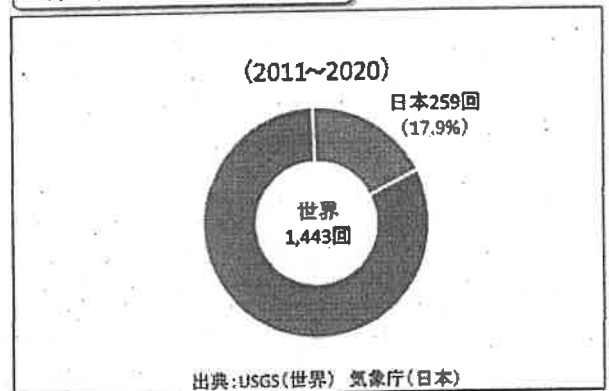
マグニチュード6.0以上の地震回数
