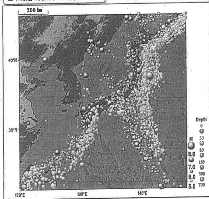
日本付近で発生した地震の分布図
